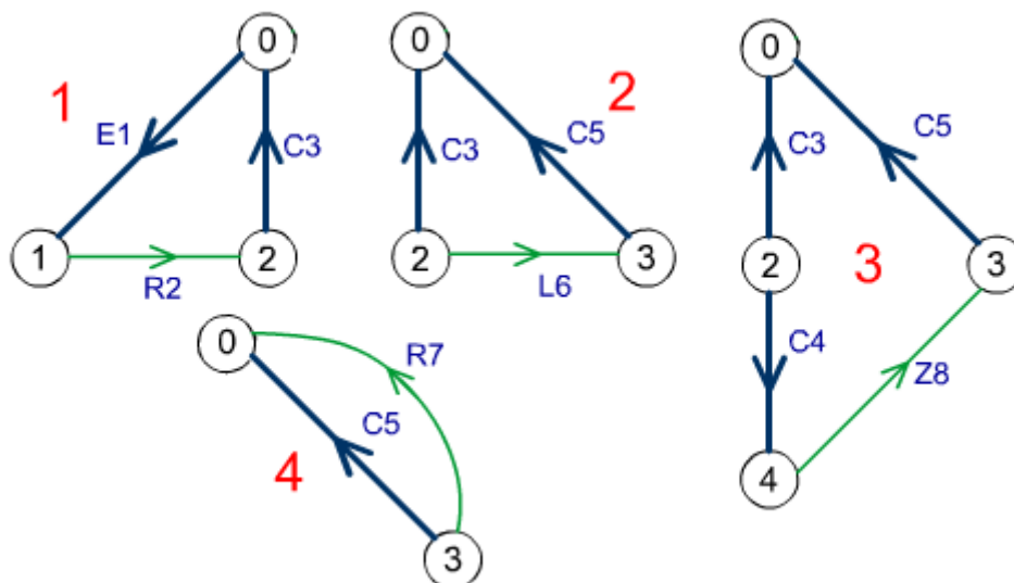
Рисунок 7. Выделение контуров.
